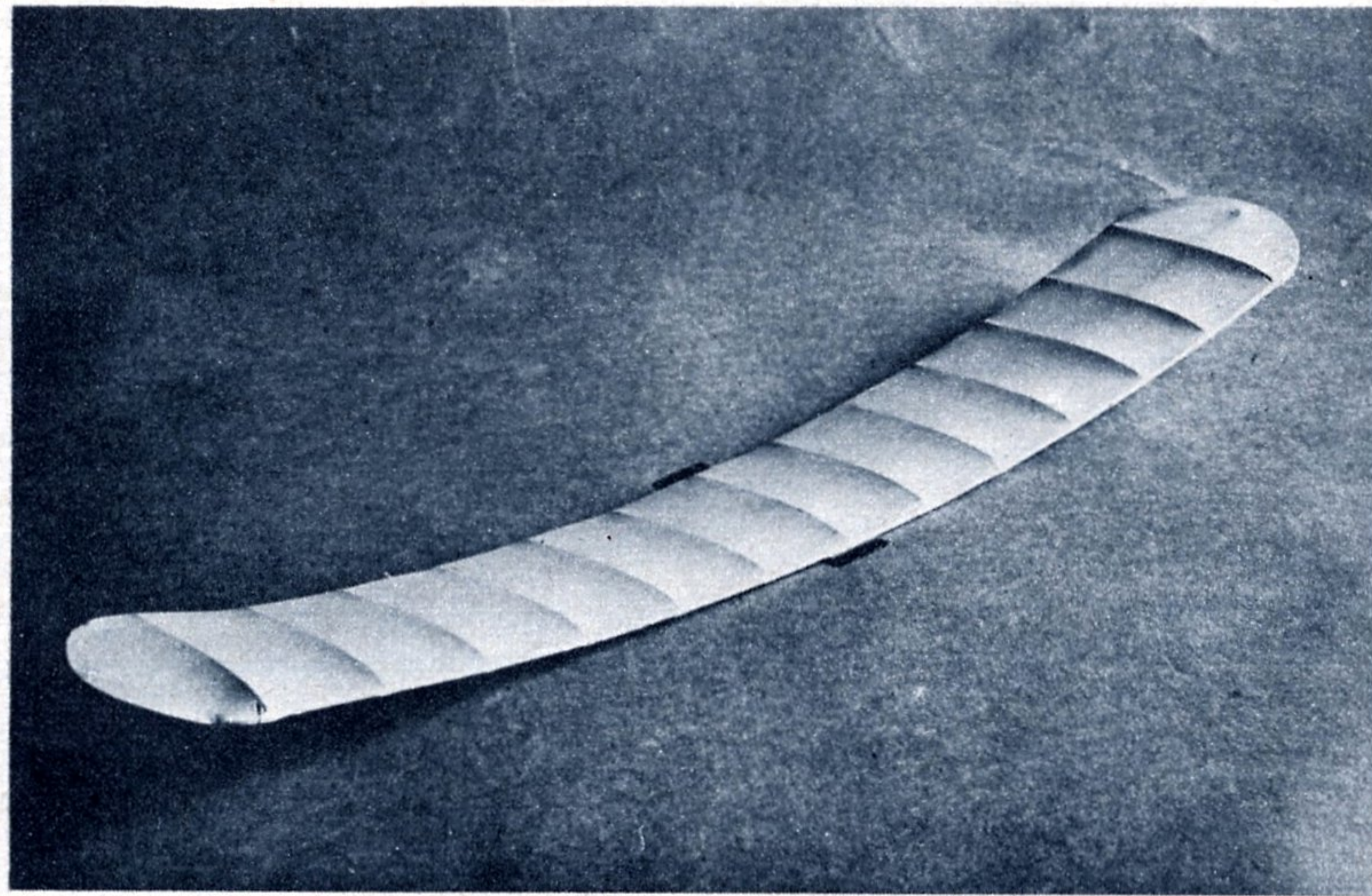
Die Tragfläche unseres Holzmodells nach dem Bespannen. Deutlich ist die gebogene Form zu erkennen Aufnahme Scherl
