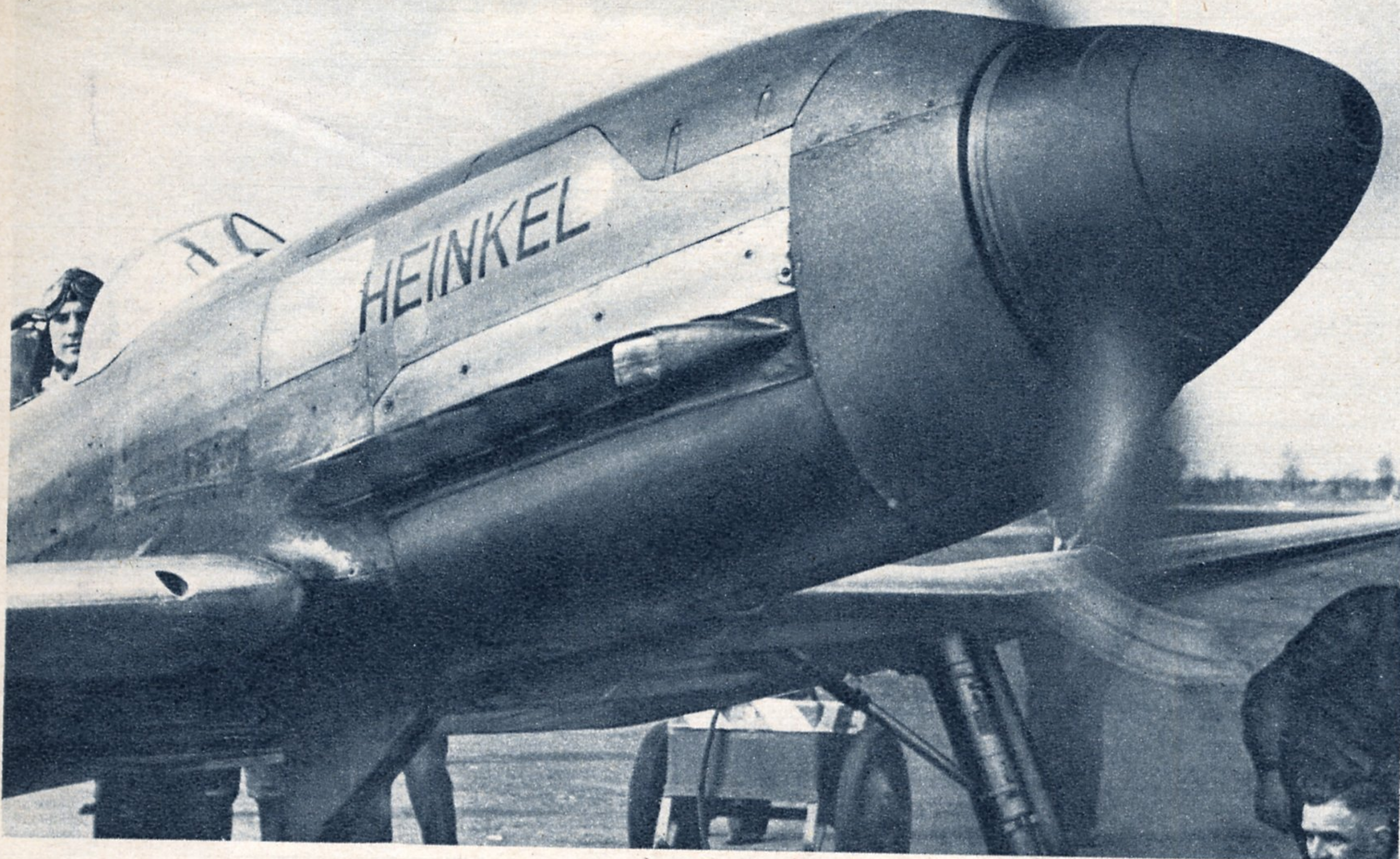
Das Flugzeug, mit dem Flugkapitän Dieterle zum schnellsten Mann der Welt wurde. Die besondere Leistung besteht darin, daß alle bisherigen Rekorde mit Wasserflugzeugen, der Dieterles aber mit einem Landflugzeug erreicht wurde
